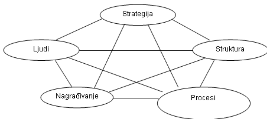
Slika 1: Model zvezda
